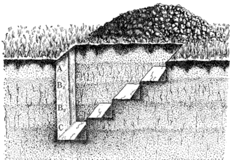
Рис. 1. Почвенный разрез
