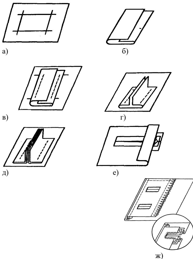
Рис. 10. Обработка обтачных петель: а) разметка петель; обработка обтачной петли одной обтачкой: б) обработка обтачки; в) притачивании обтачки; г) выправление срезов обтачки; обработка обтачной петли двумя обтачками: д) притачивание обтачек; е) закрепление уголков петли; ж) обработка петли со стороны подборта.
