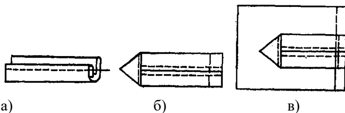
Рис. 13. Петля из прямой полоски ткани: а) застрачивание полоски для петли; б) образование треугольника; в) притачивание петли к детали.
